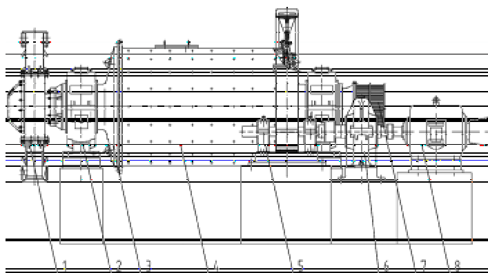
1. 联合轴衬 2. 轴承 3. 进料部 4. 筒体 5. 传动部 6. 减速机 7. 出料部 8. 电动机
